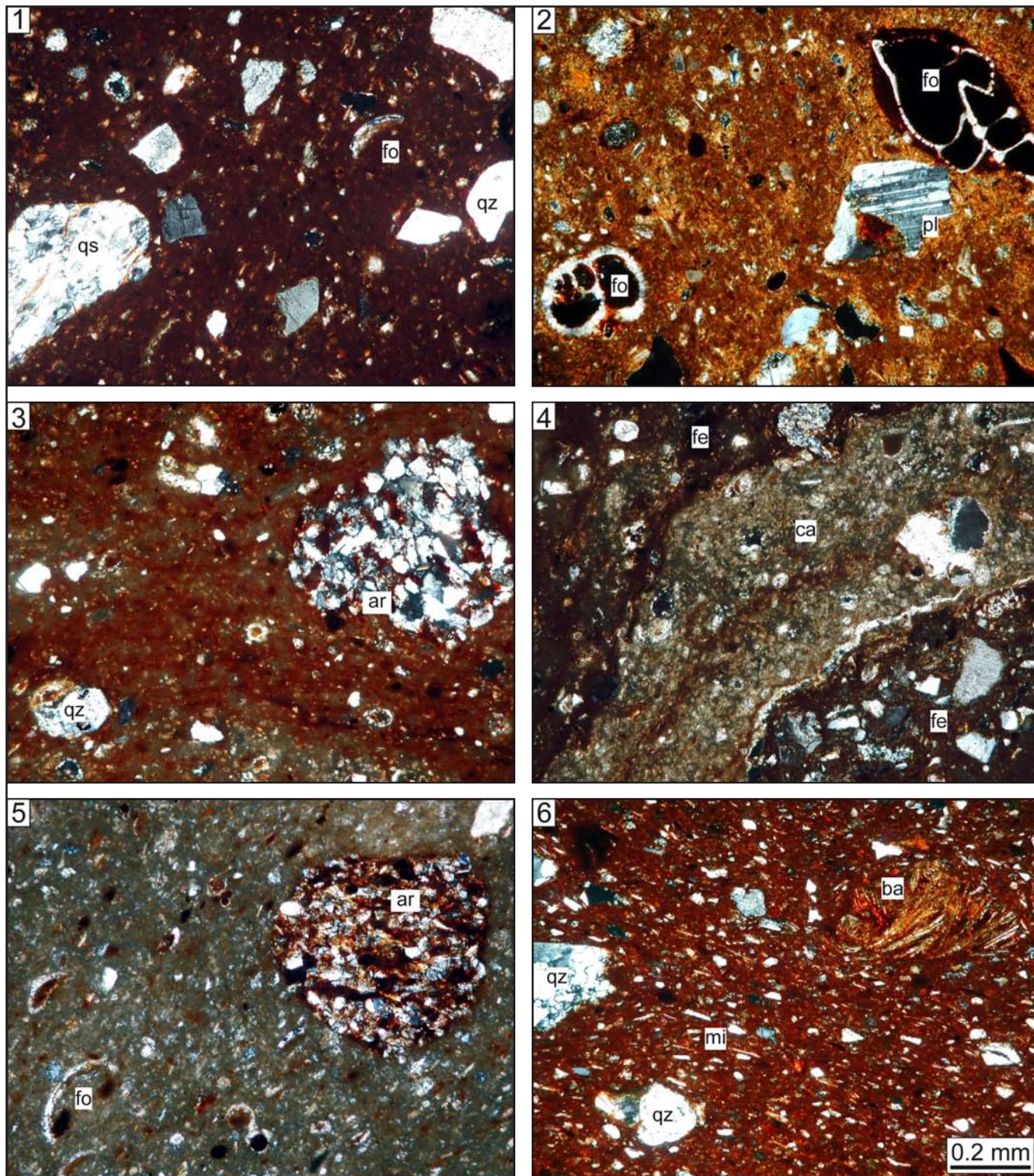
Pl. hors-texte 16 : Particolari in sezione sottile (nicol incrociati) di alcuni campioni rappresentativi. 1: 7831, 2: 7838, 3: 7832, 4: 7836, 5: 7834, 6: 7833; ar: arenite, ba: basalto, ca: argilla carbonatica, fe: argilla ferrica, fo: fossile calcareo, mi: mica, pl: plagioclasio, qs: quartzoscisto, qz: quarzo.
